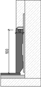
СКРЫТЫЙ ПЛИНТУС
